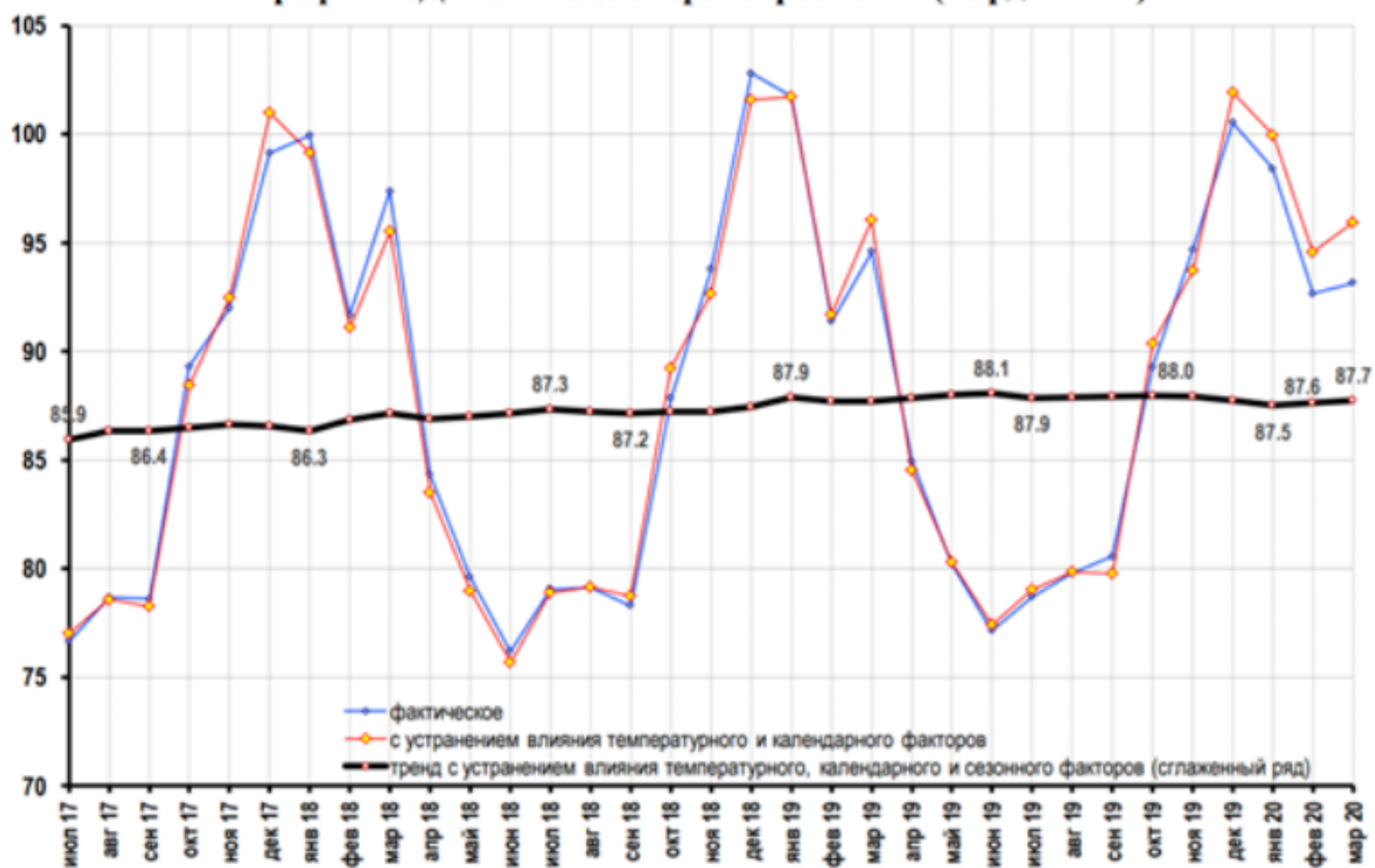
График 1. Динамика электропотребления (млрд. кВт·ч)
